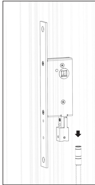
Das Umlenkschloss mit dem Anschlussstück auf das obere Ende der Treibriegelstange stecken.
