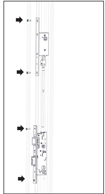
Beide Schlösser mit den Stulpschrauben anschrauben.
