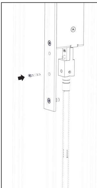
Im Anschluss mit einem SW2,5 Sechskant durch die untere kleine Stulpbohrung das Anschlussstück an die Treibriegelstange fest anschrauben.
