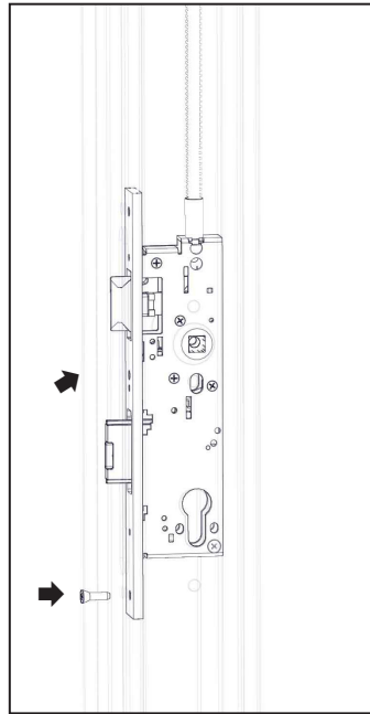
Hauptschloss (mit eingedrehter Treibriegelstange) einstecken und untere Stulpschraube zur Hälfte eindrehen.
