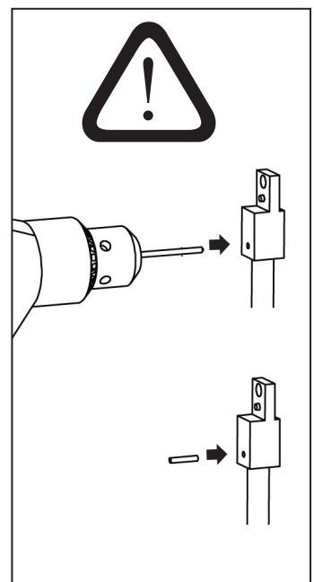
Durchgangsbohrung D= 2,5mm komplett durch Anschlussstück und Stange bohren. Spannstift bündig eintreiben.
