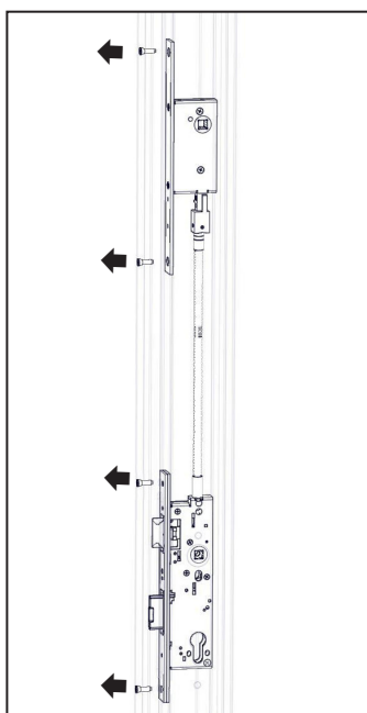
Die Stulpschrauben beider Schlösser werden gelöst, die Schlösser entnommen.
