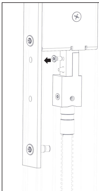
Mit einem SW2,5 Sechskant das Anschlussstück vom Umlenkschloss abschrauben.
