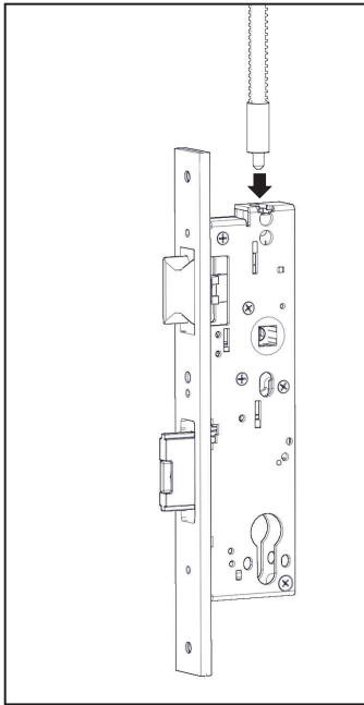
Treibriegelstange handfest in das Hauptschloss eindrehen.
