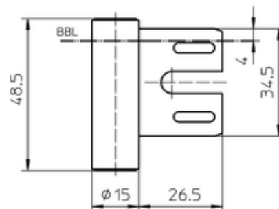
Vorderansicht
