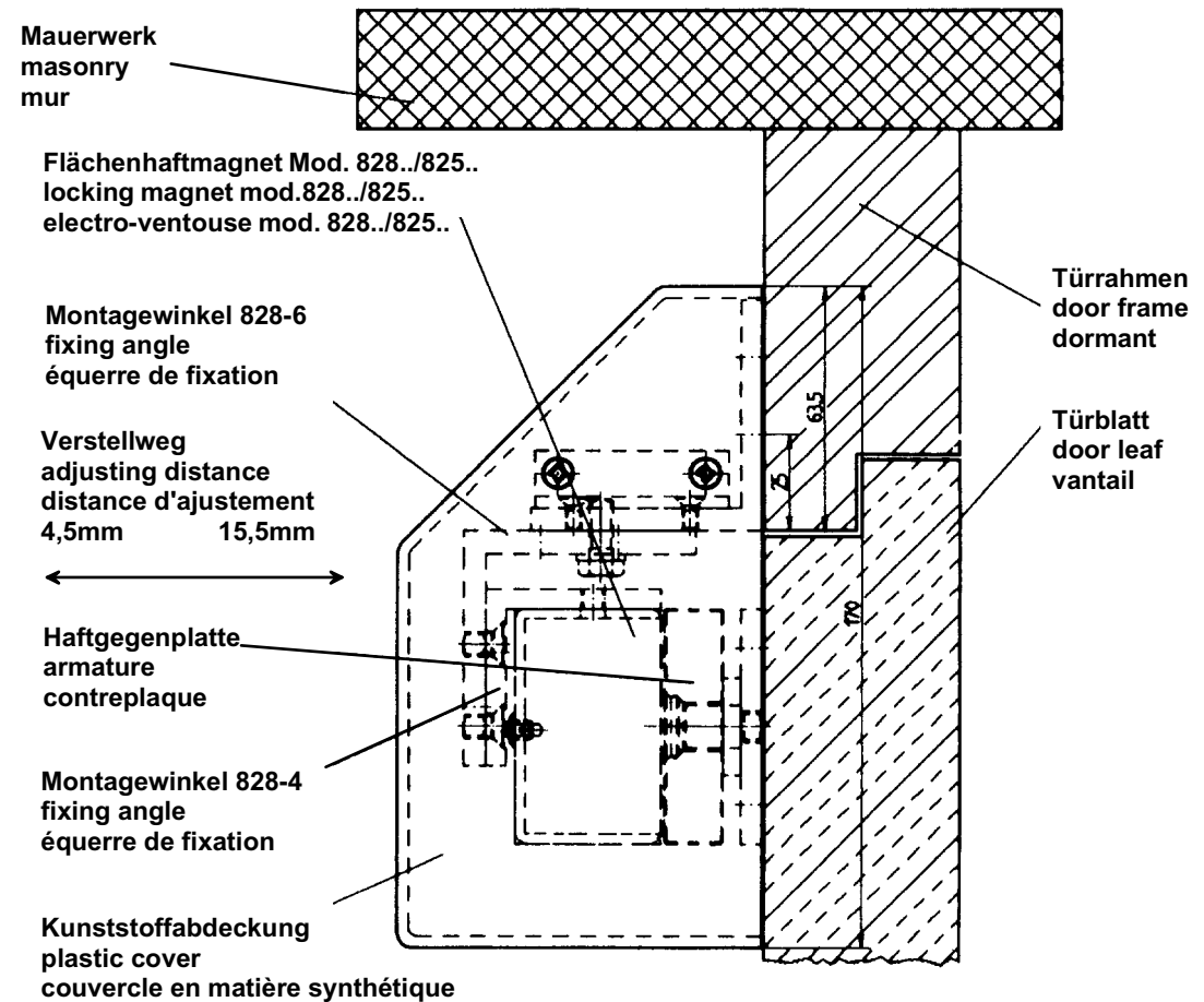
Version "B": Nach außen öffnende Tür door opening outwards porte s'ouvrant vers l'extérieur
