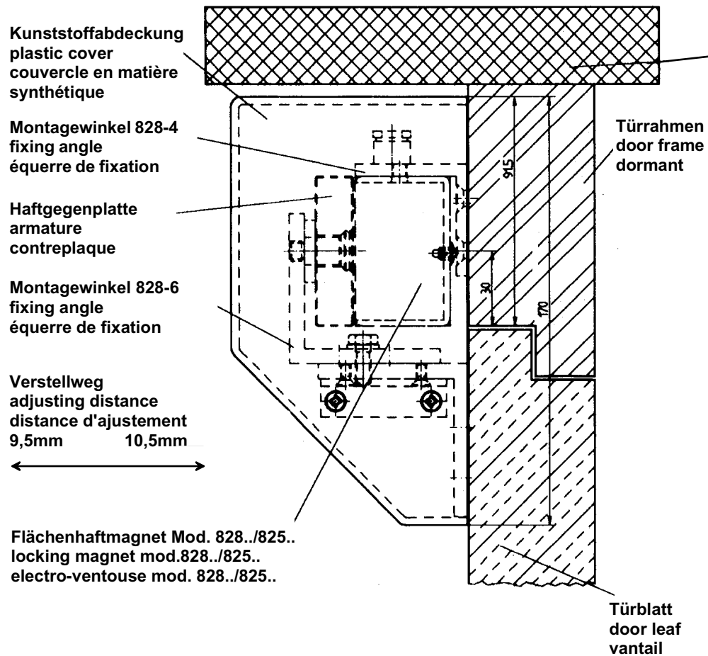
Version "A": Nach innen öffnende Tür door opening inwards porte s'ouvrant vers l'intérieur
