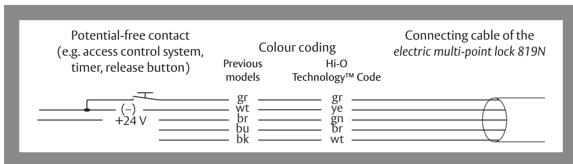
Fig. 13: Wiring diagram
