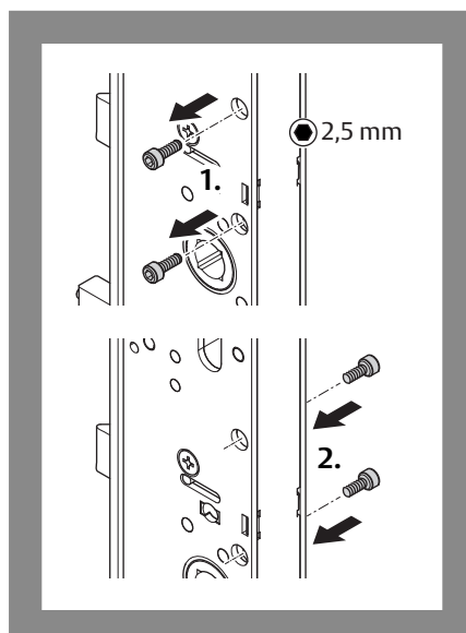
Fig. 12: Regolazione del lato antipanico
