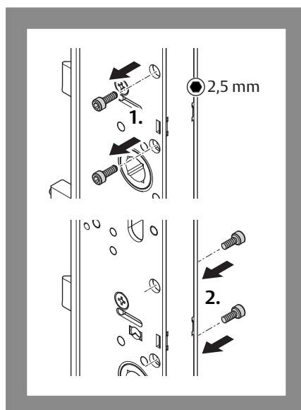
Afb. 12: Paniekzijde instellen
