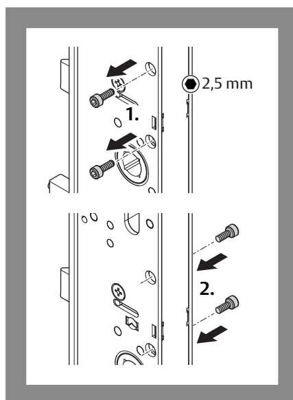
Abb. 12: Panikseite einstellen
