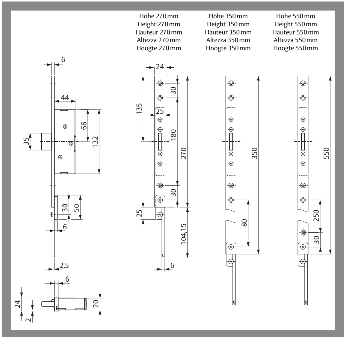
Abb. 27: Abmessungen Zusatzriegel
