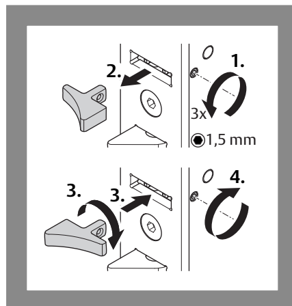
Afb. 9: Stuurschoot draaien
