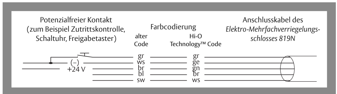
Abb. 13: Anschlussplan
