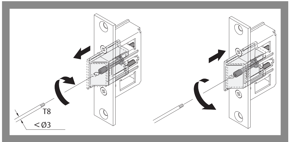
Afb. 11: Schootuitslag van schootslot 807-10 instellen
