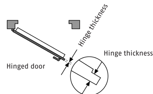
DIN right
