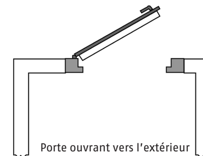
Porte affleur
