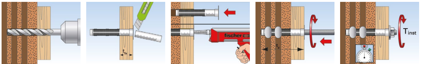
Lochstein (Durchsteckmontage)
